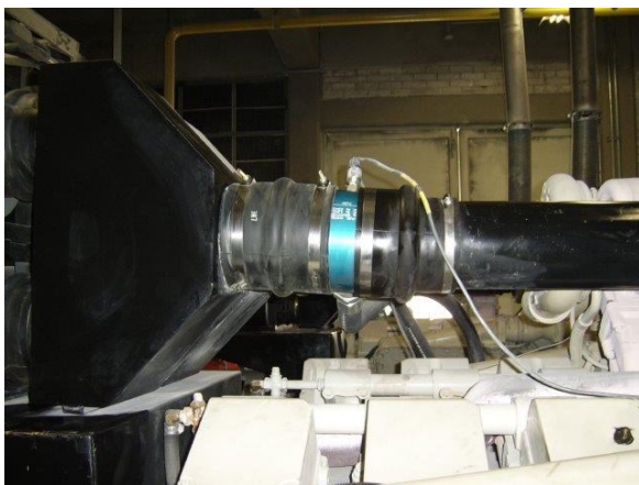
Mezclador de gas después de filtros de aire
